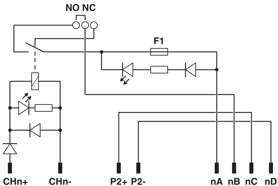
Schaltplan
