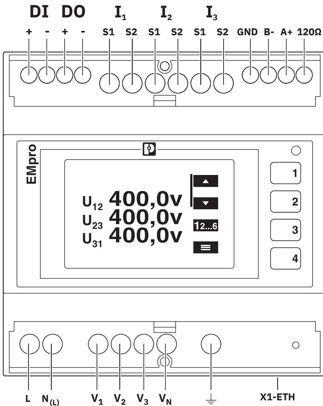
Anschlusszeichnung
