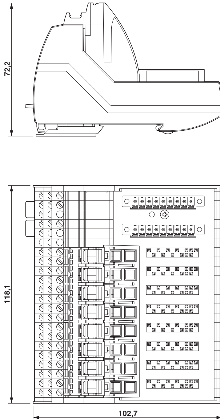
Maßzeichnung
