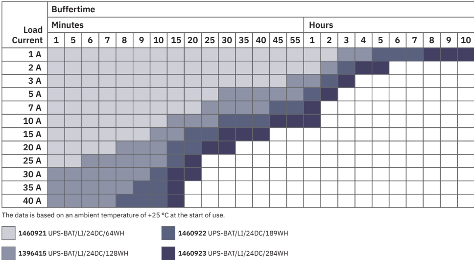
Pufferzeiten QUINT DC-USV für LI-Batteriemodul
