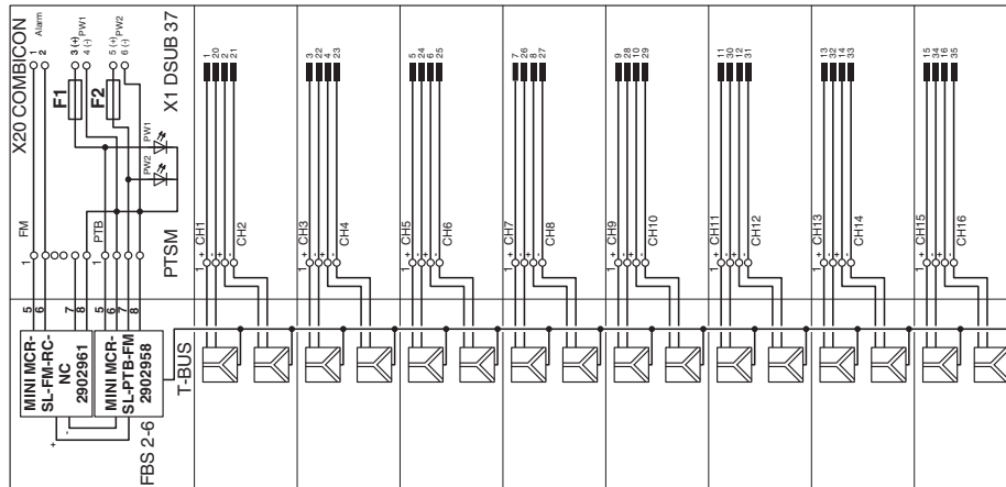
Schaltplan
