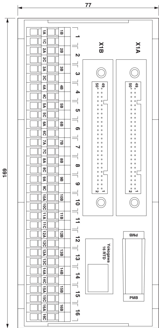
Maßzeichnung
