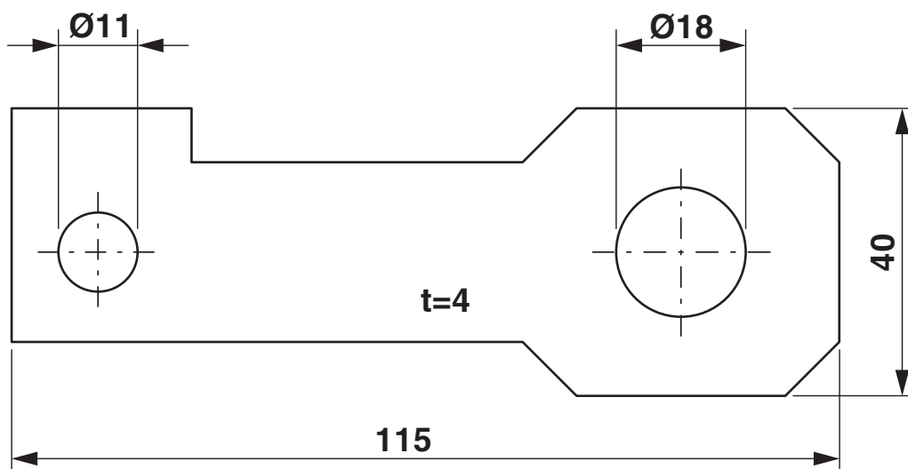
Maßzeichnung
