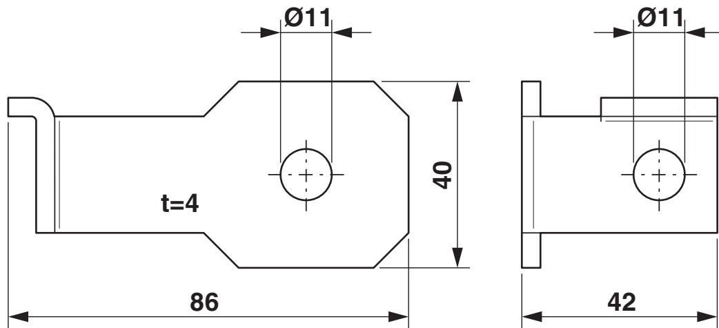
Maßzeichnung
