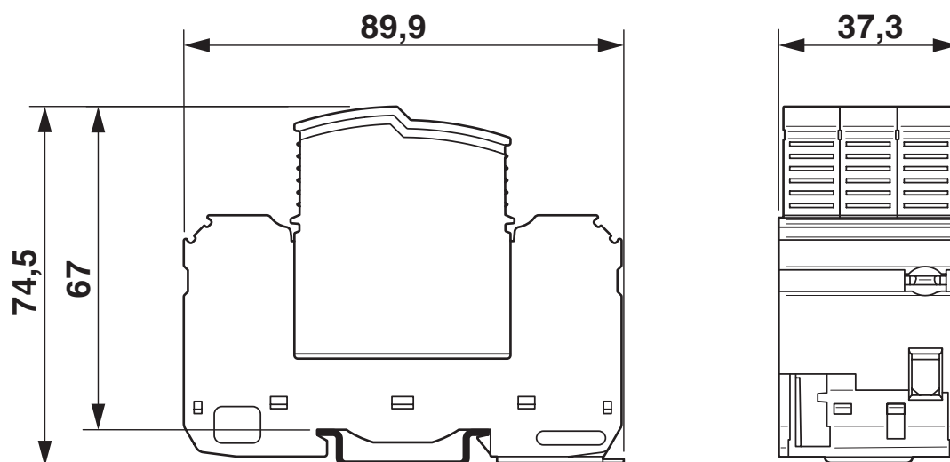
Maßzeichnung
