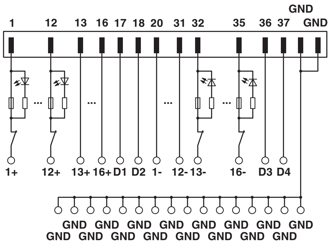
Schaltplan
