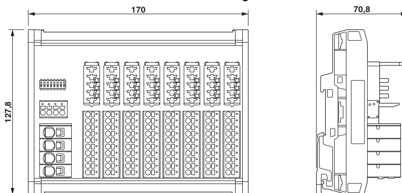
Maßzeichnung
