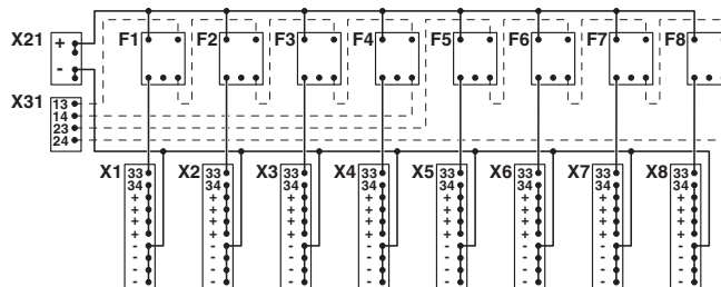
Schaltplan
