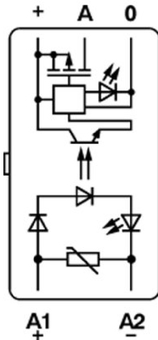
Schaltplan
