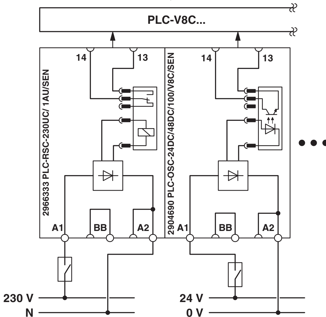
Schaltplan
