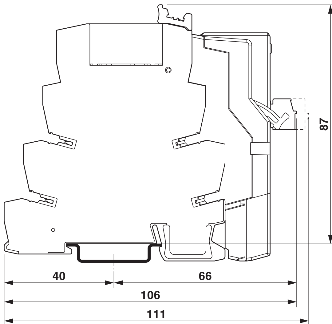
Maßzeichnung
