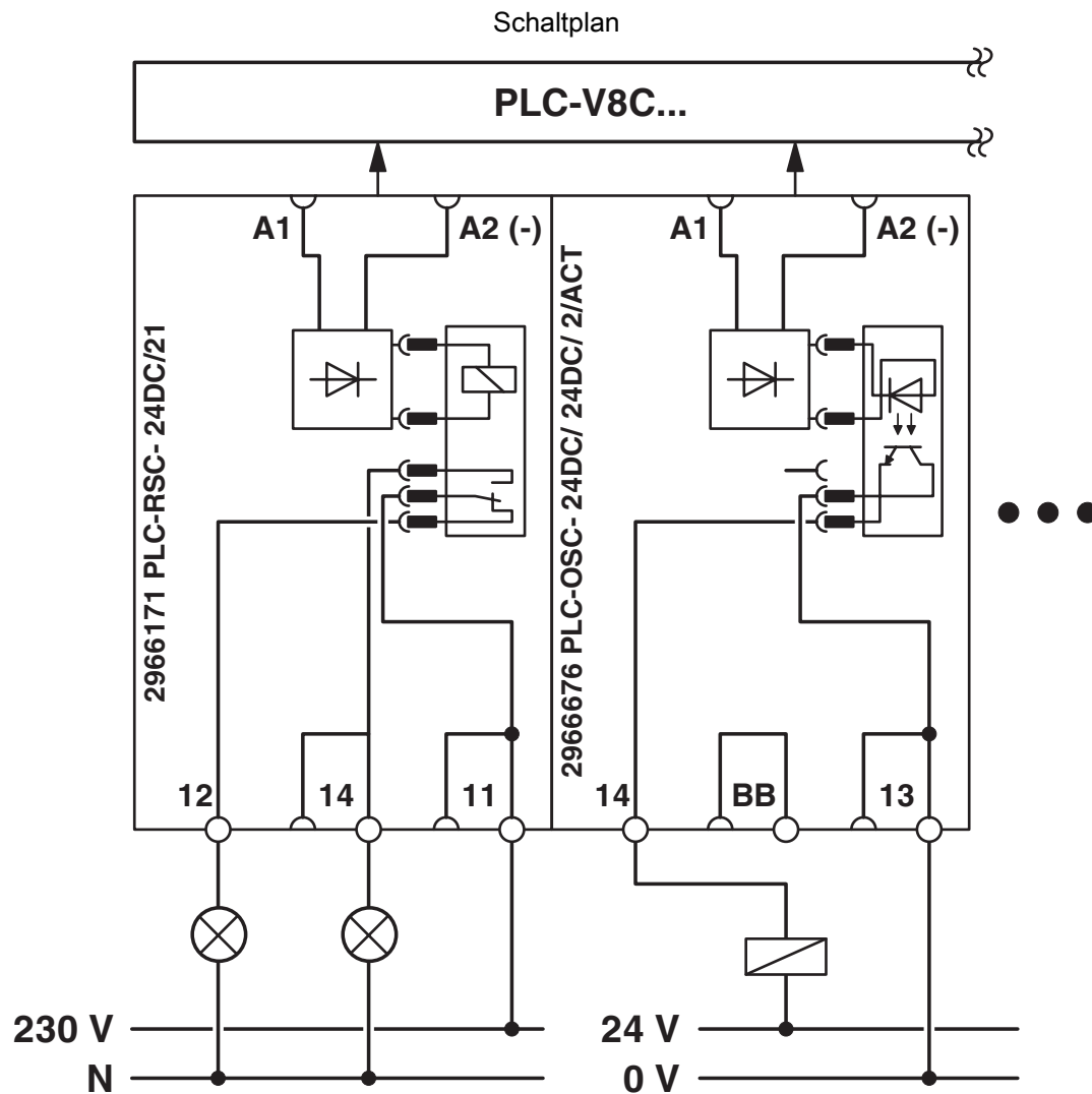
Prinzipialschaltplan: Ausgänge über PLC-INTERFACE am Beispiel einer Ausgabeklemme mit Relais, 1 Wechsler und einer Ausgabeklemme mit Solid-State Relais.
