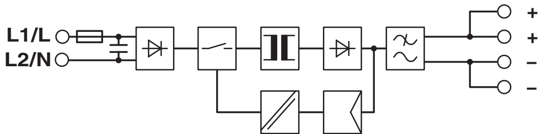
Blockschaltbild
