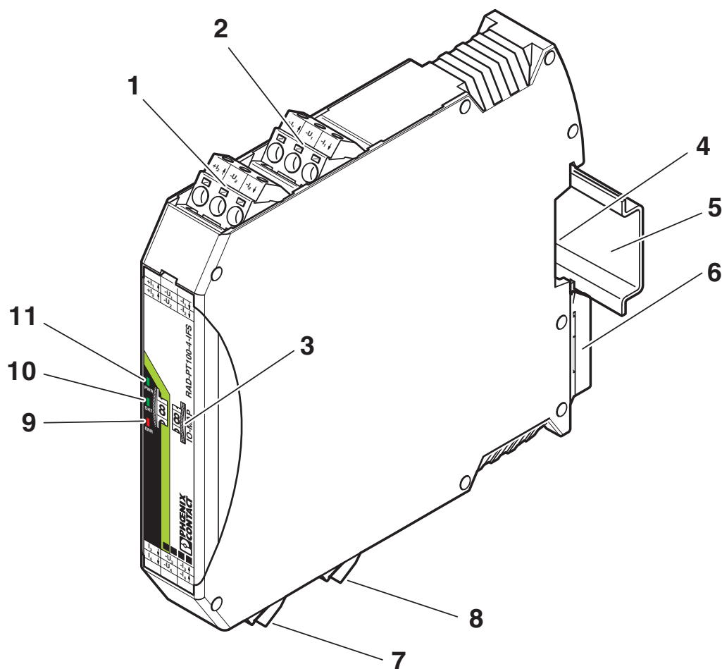
Schemazeichnung
