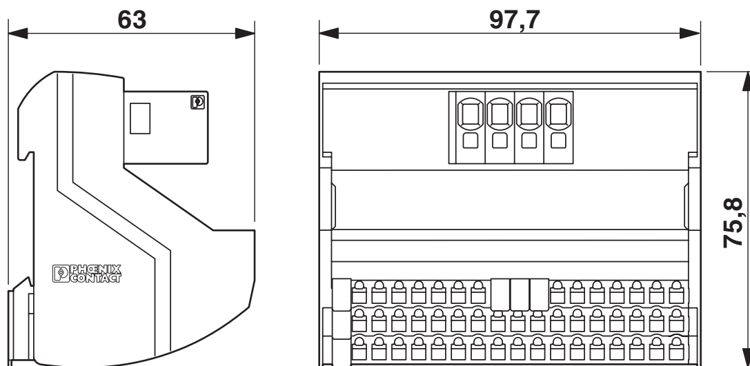
Maßzeichnung
