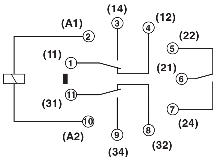
Schaltplan
