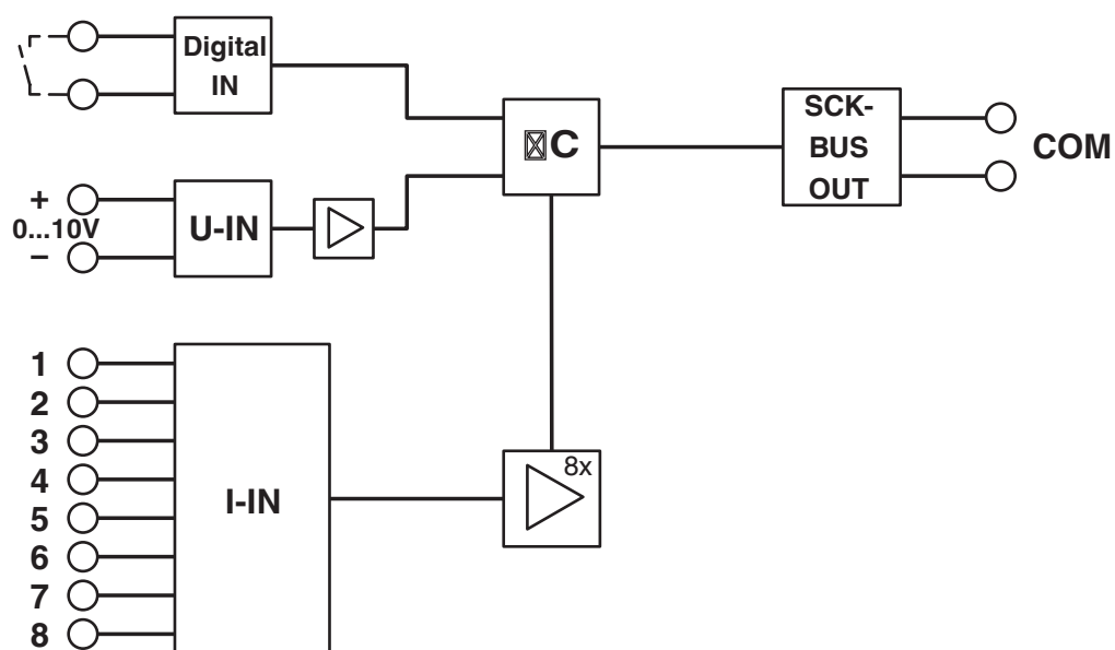
Blockschaltbild
