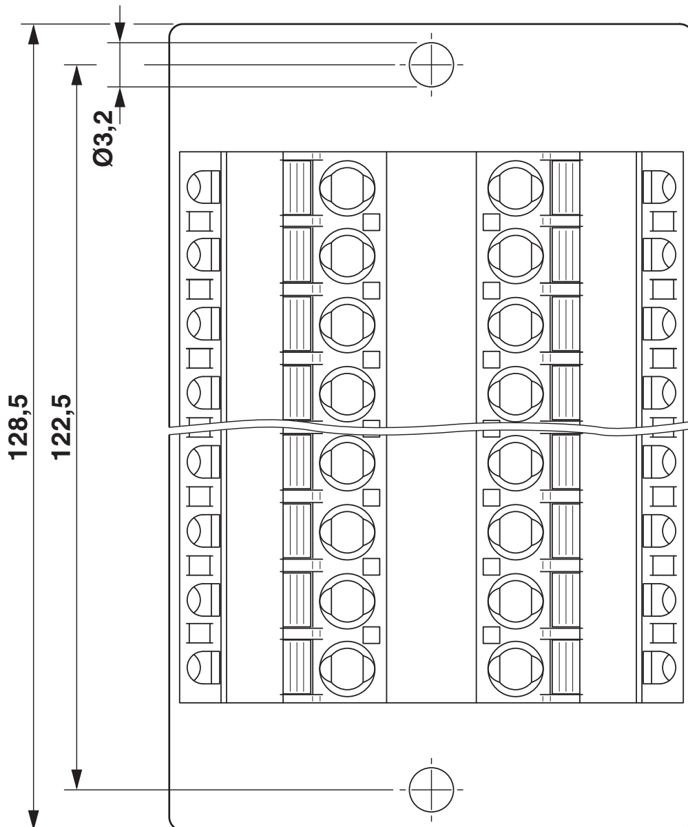
Maßzeichnung
