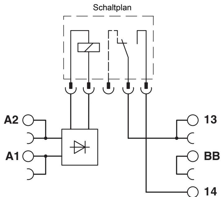
Schaltplan
