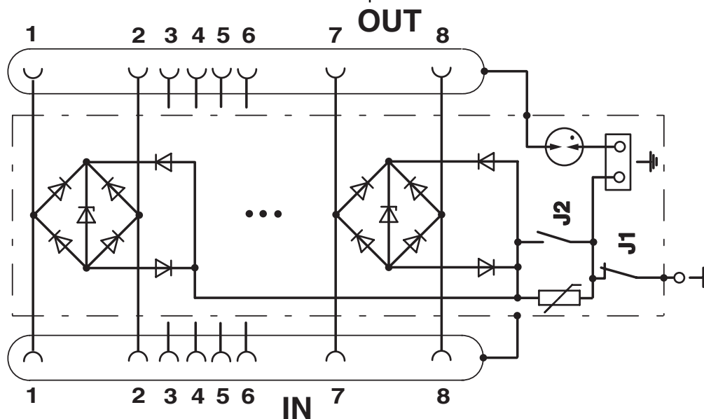
Schaltplan
