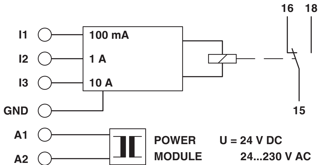
Blockschaltbild
