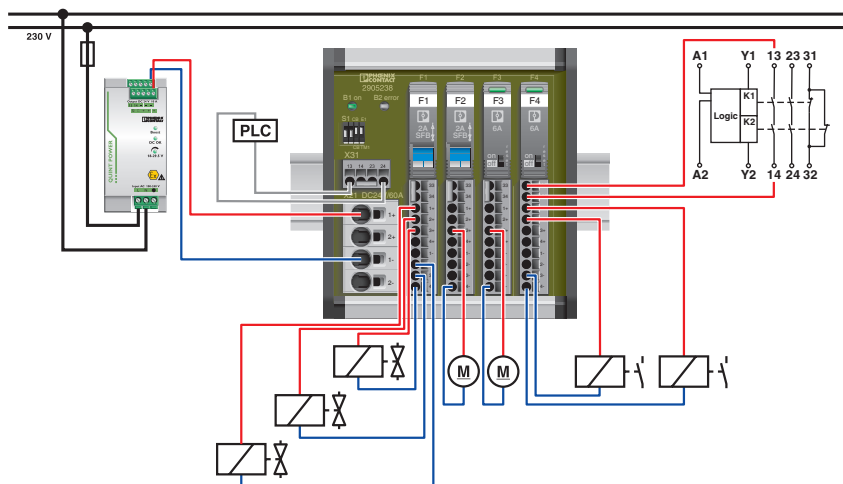
Applikationszeichnung
