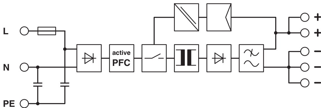
Blockschaltbild
