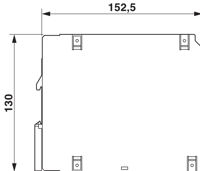
Maßzeichnung
