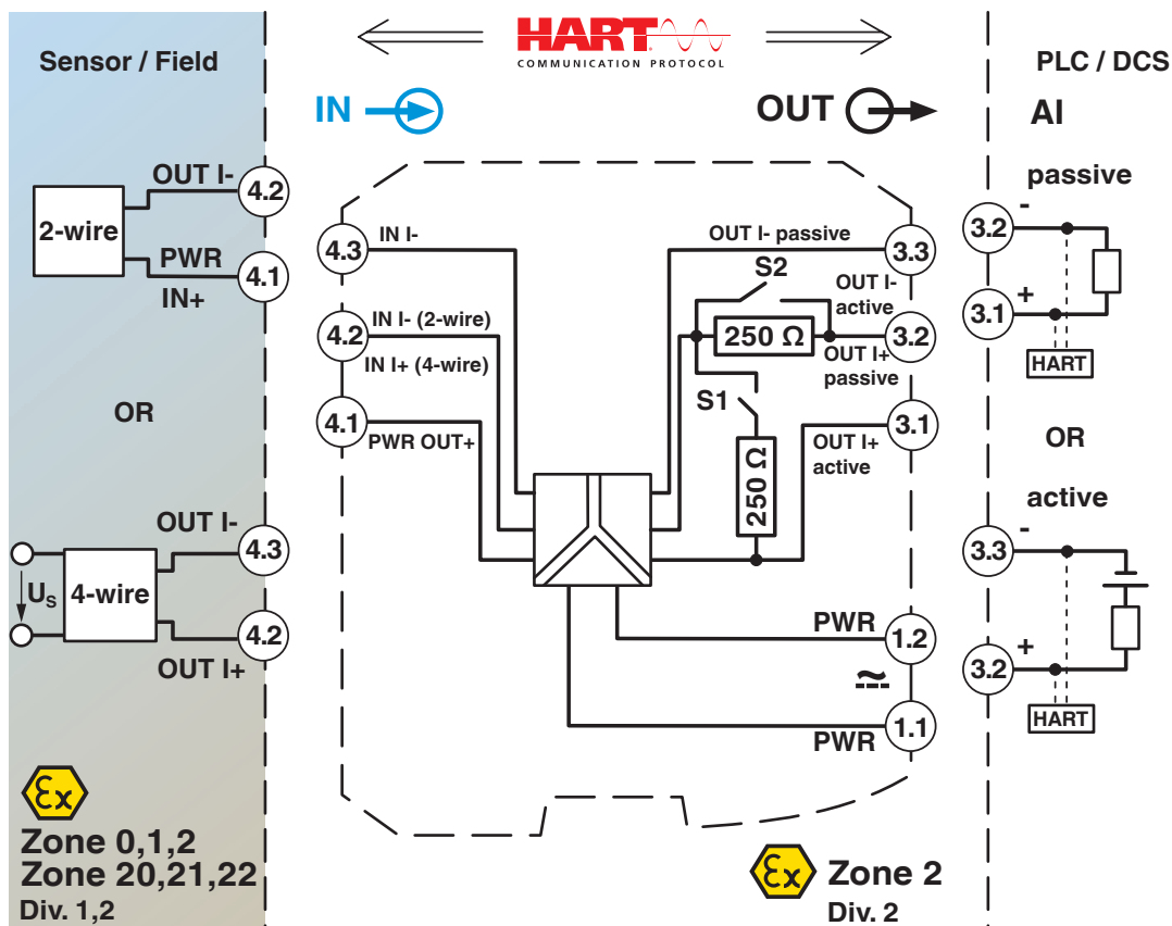
Blockschaltbild
