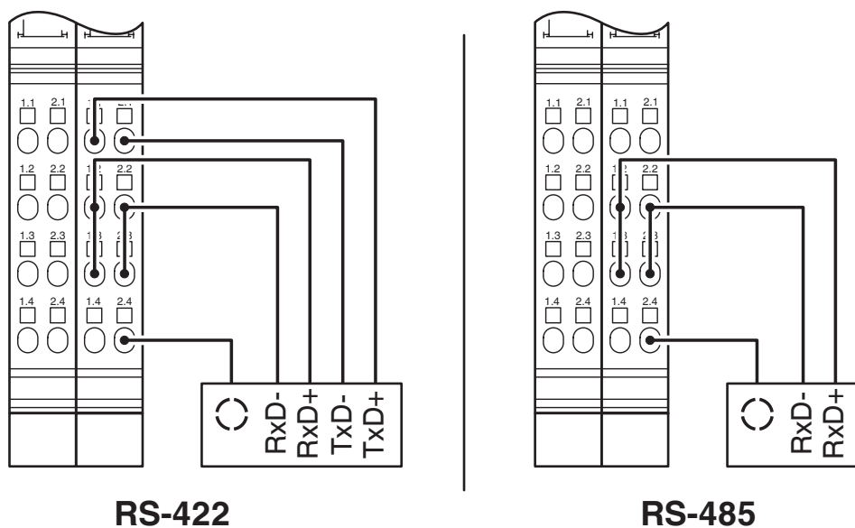
Anschlusszeichnung
