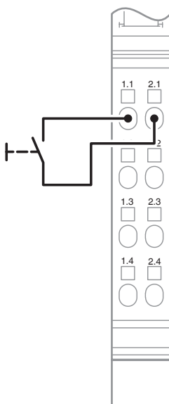
Anschlusszeichnung
