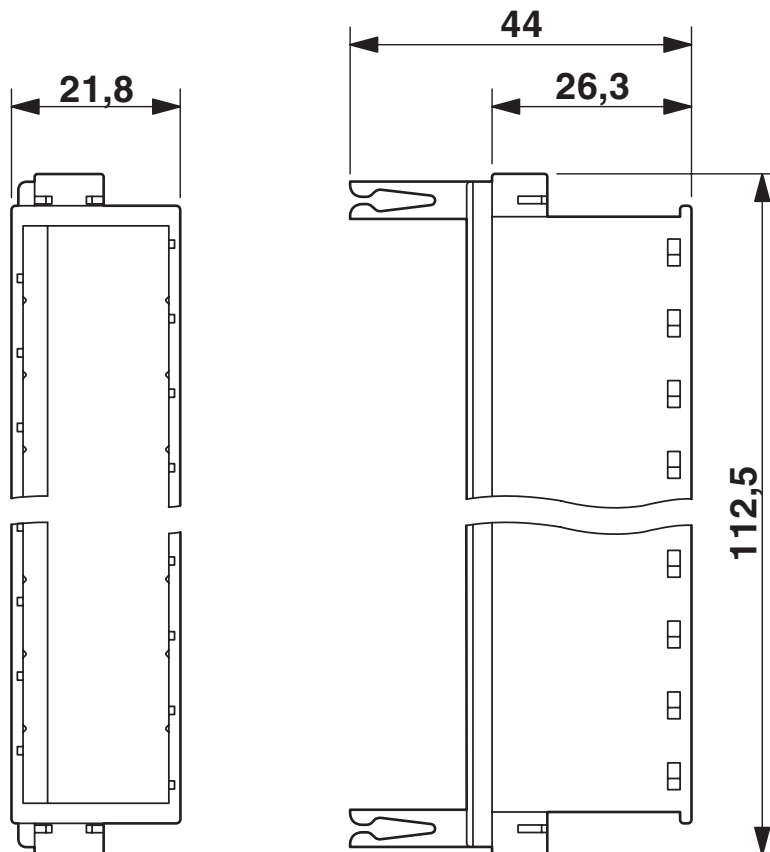
Maßzeichnung
