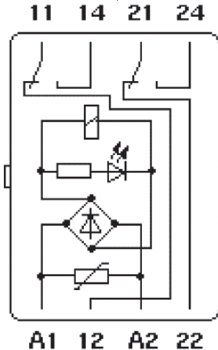
Schaltplan
