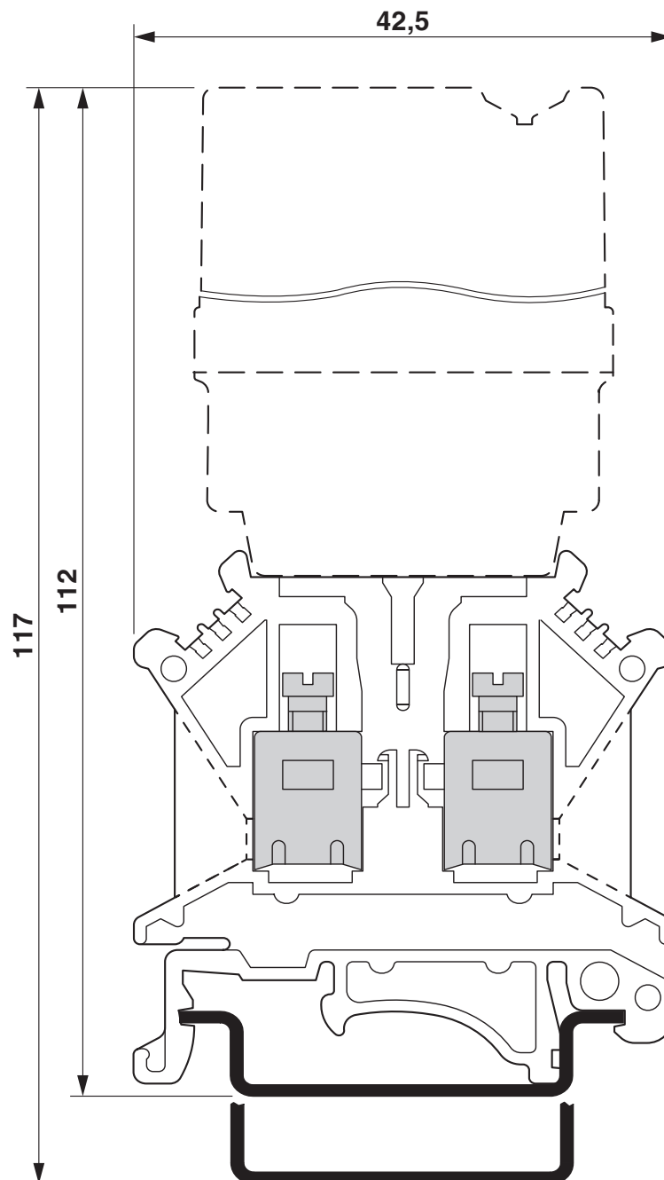
Maßzeichnung
