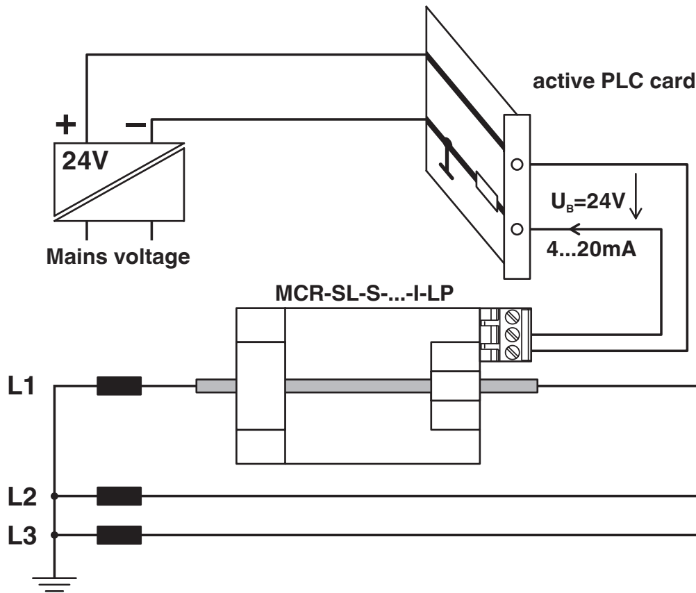
Applikationszeichnung
