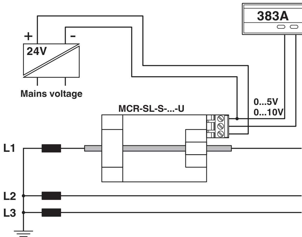
Applikationszeichnung
