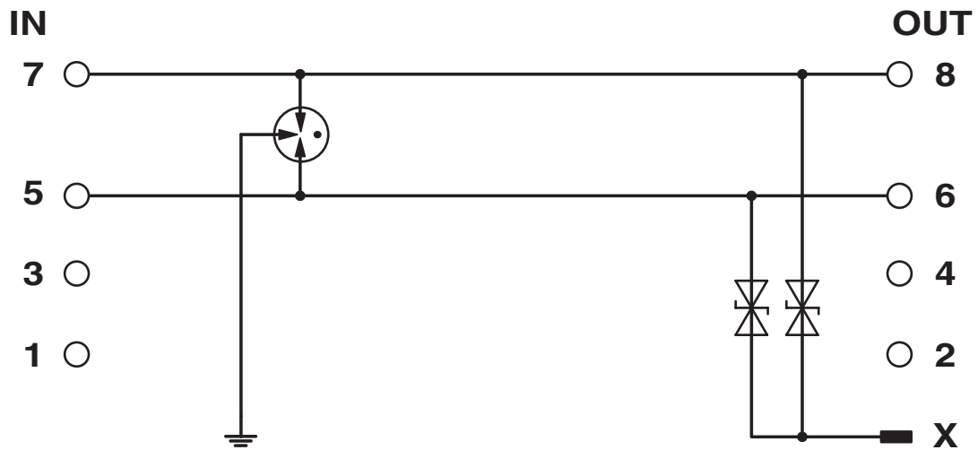
Schaltplan
