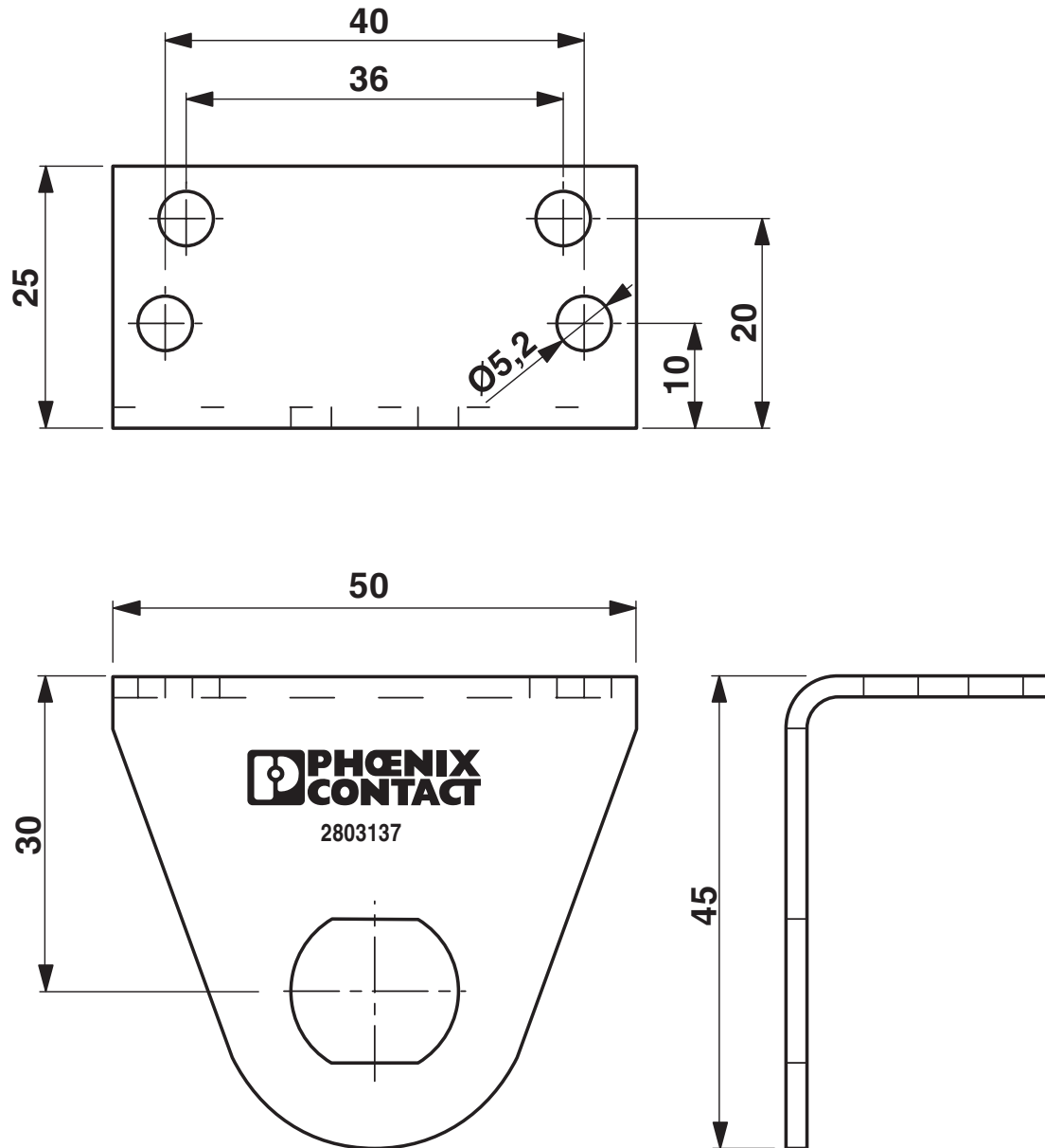
Maßzeichnung
