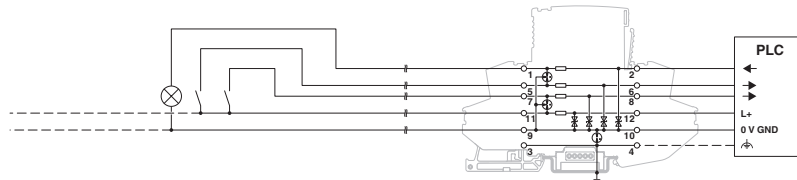
Applikationszeichnung
