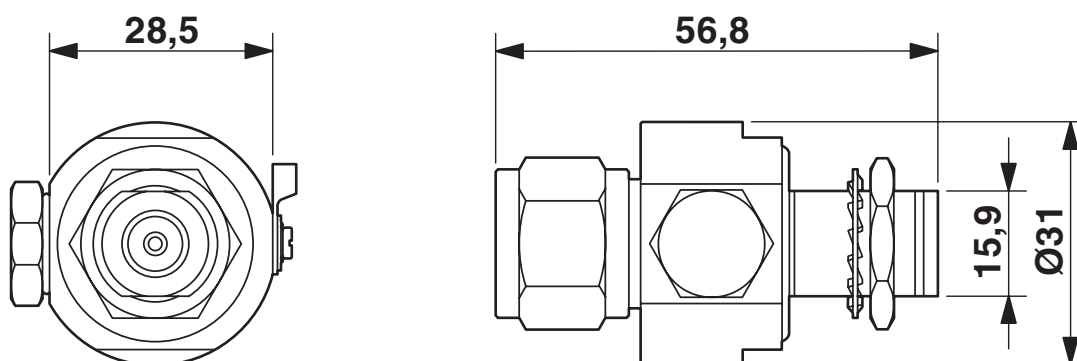
Maßzeichnung
