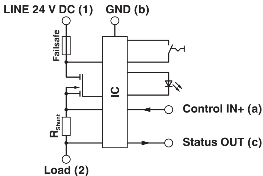
Schaltplan
