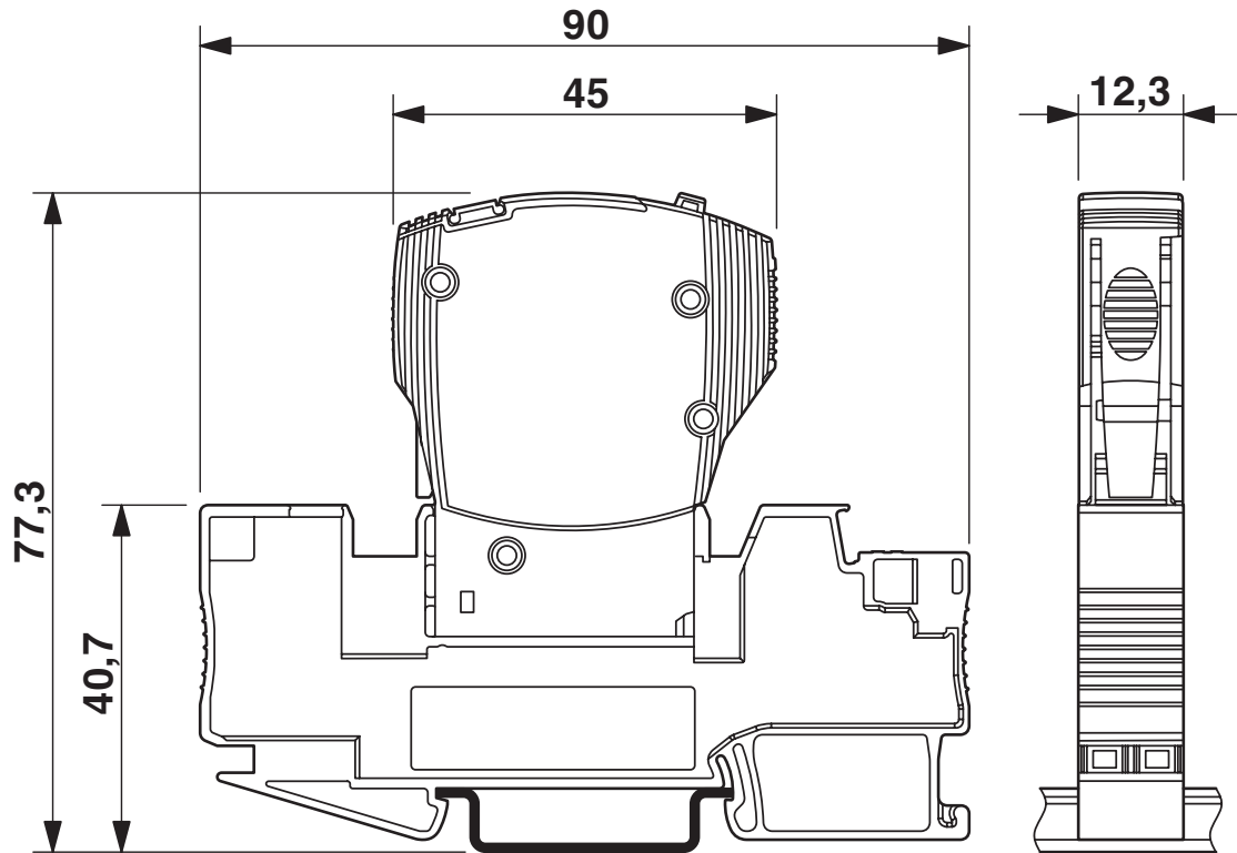
Maßzeichnung
