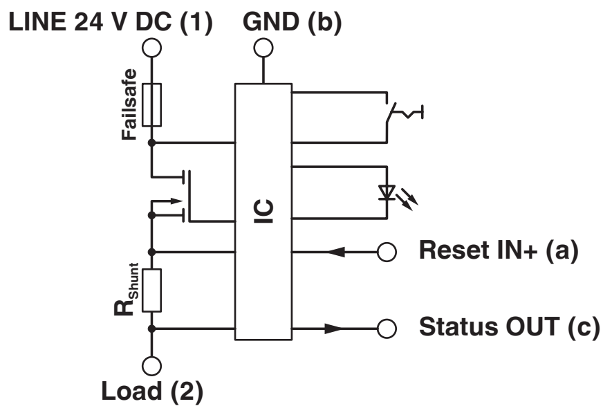
Schaltplan
