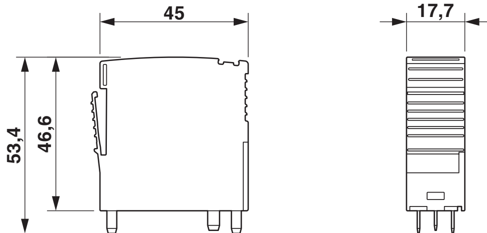
Maßzeichnung
