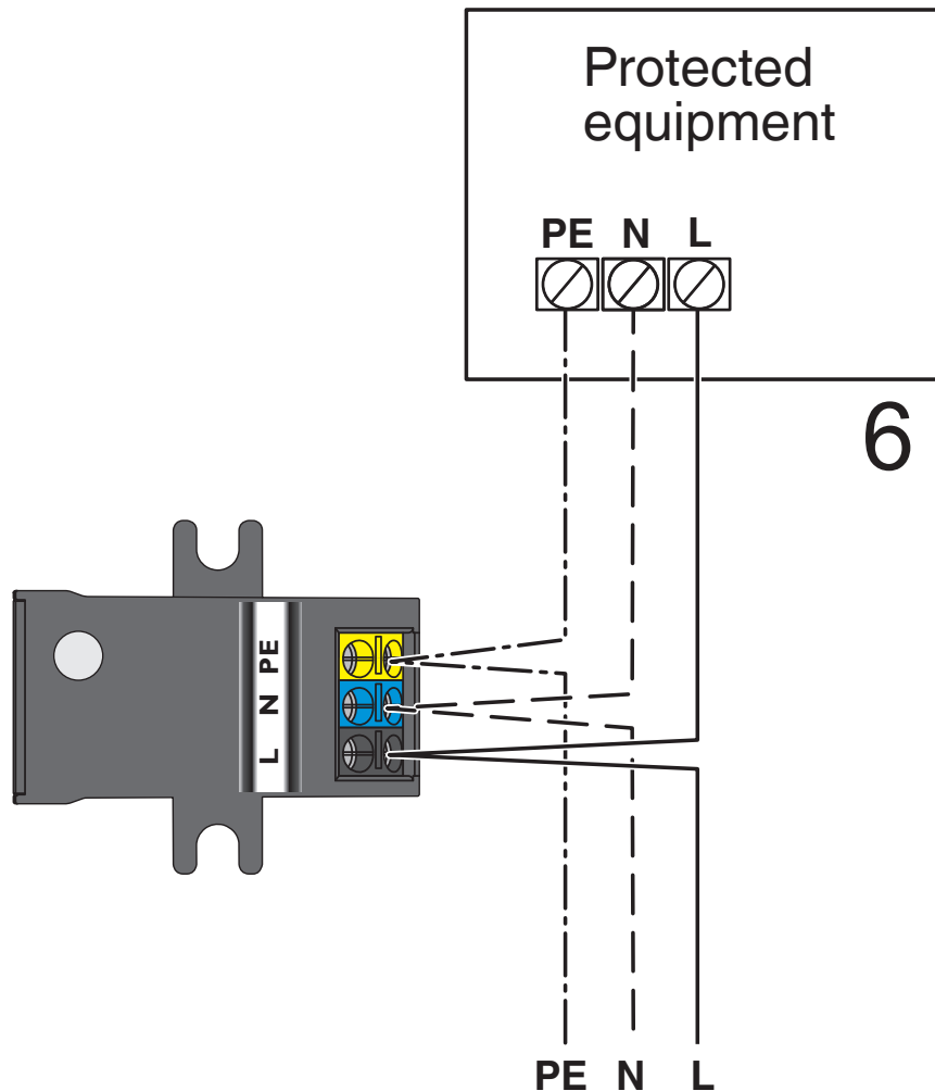
Applikationszeichnung
