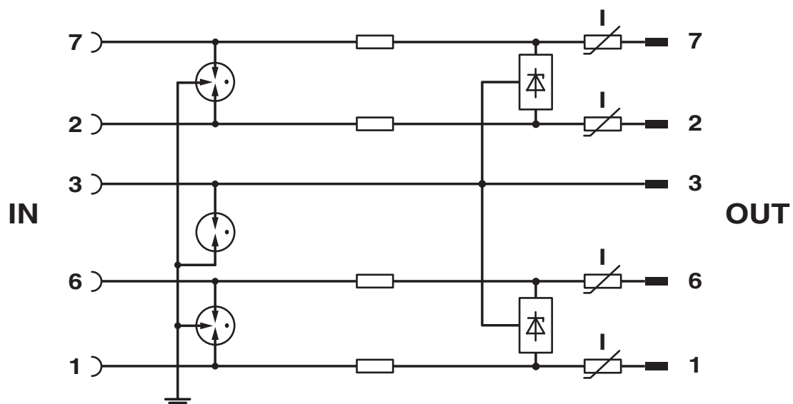
Schaltplan
