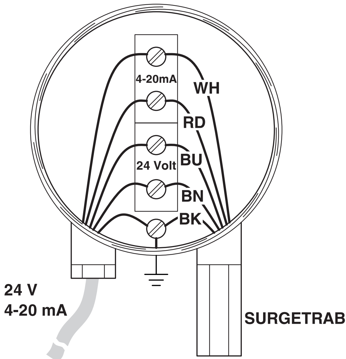
Applikationszeichnung
