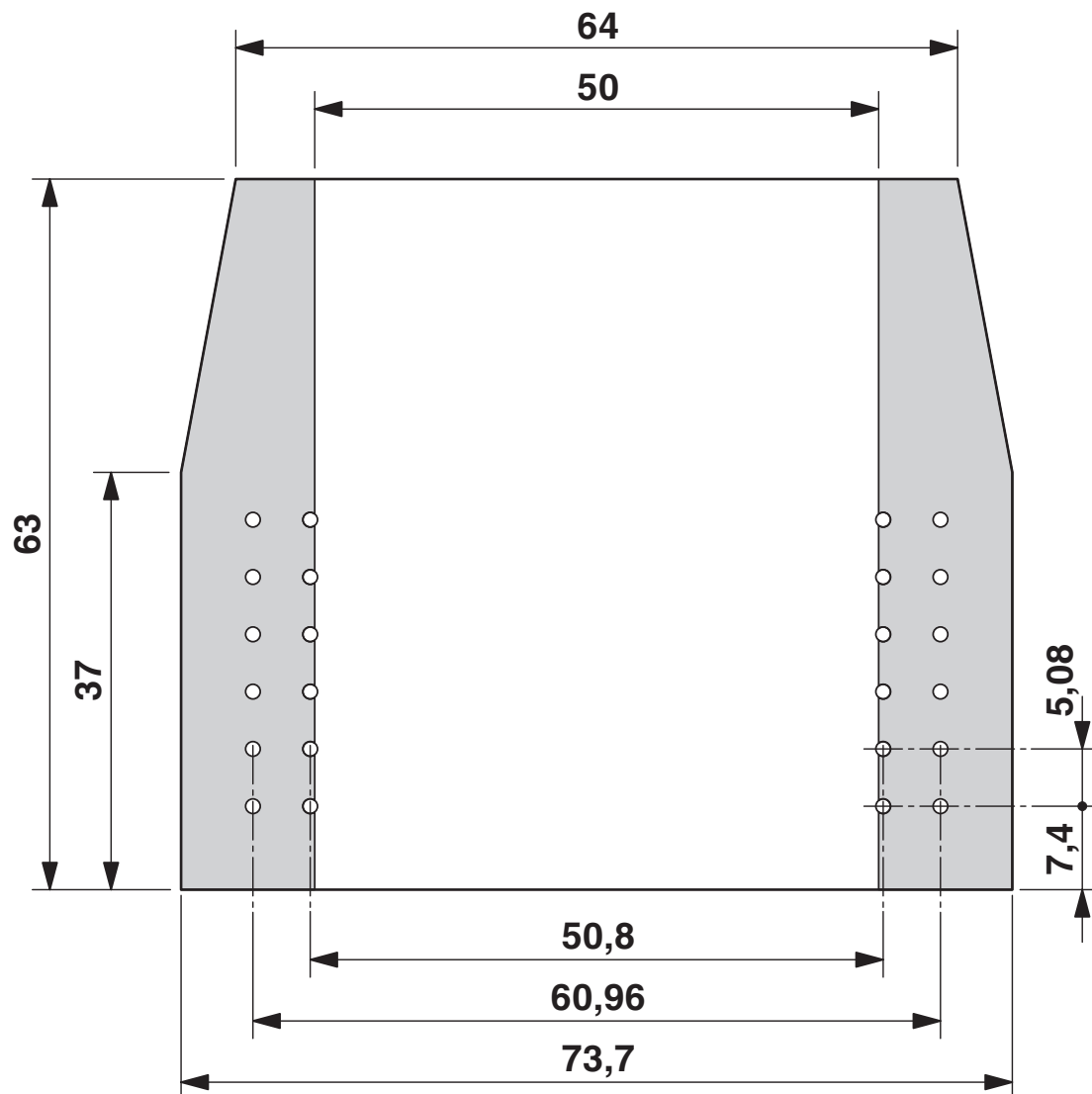
Maßzeichnung
