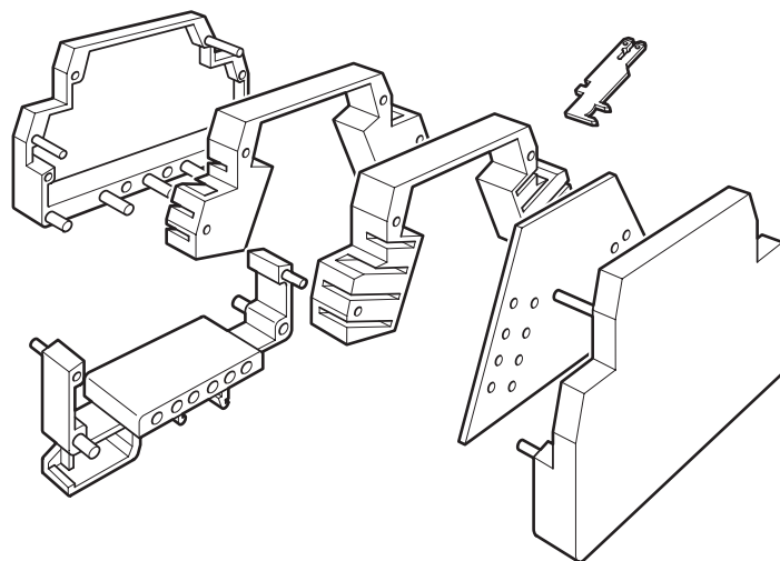
Explosionszeichnung
