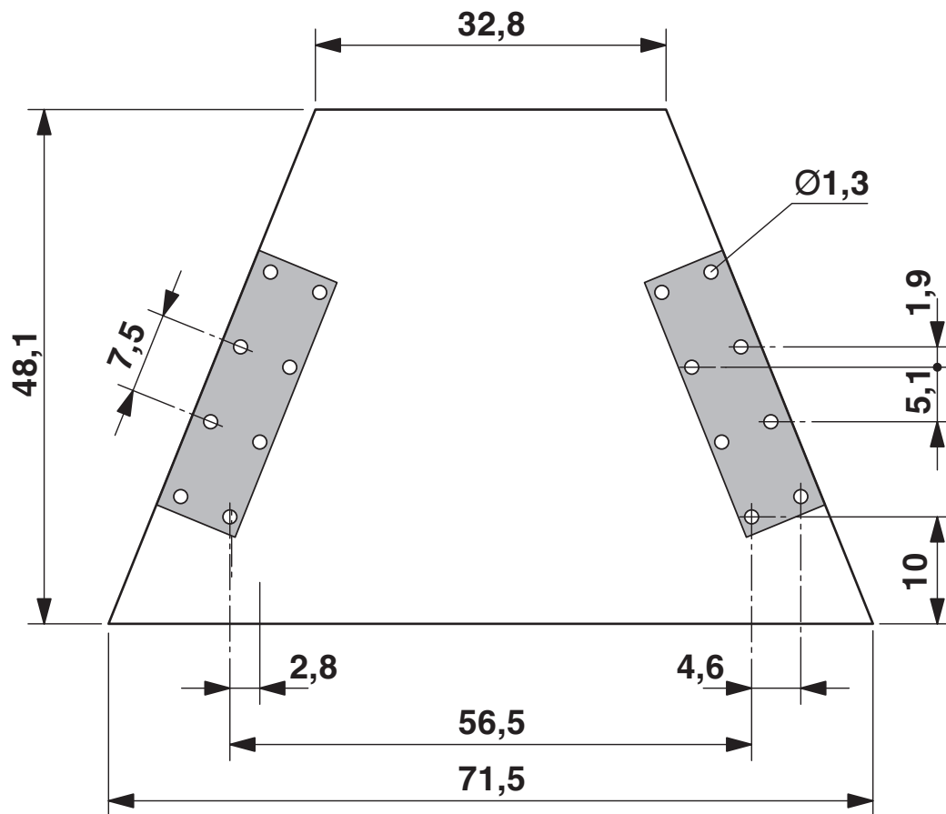
Maßzeichnung
