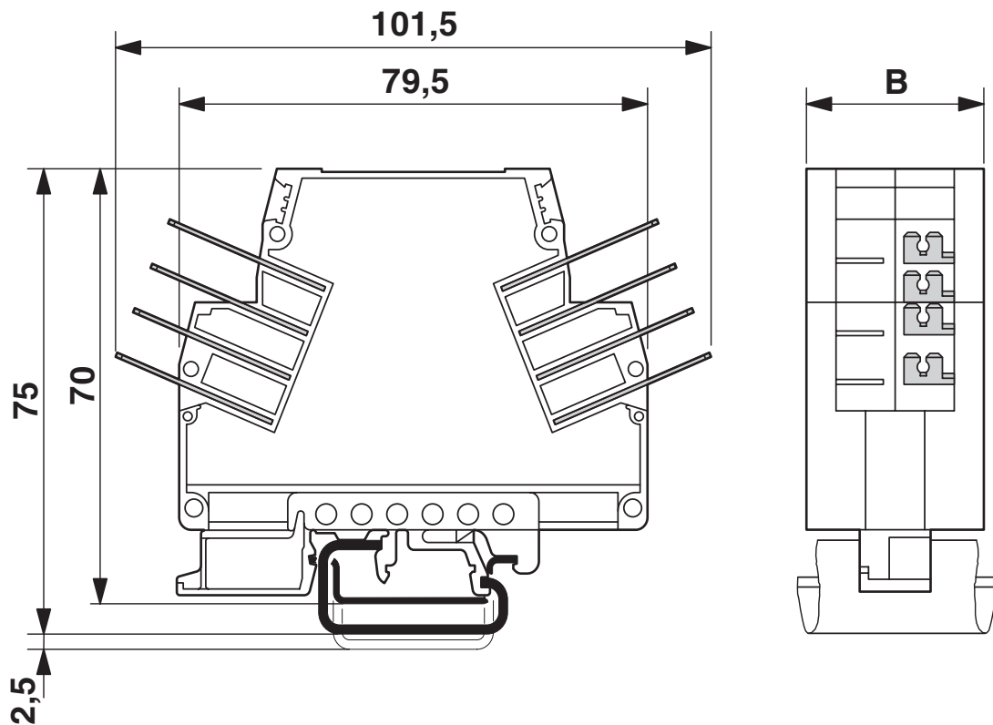
Maßzeichnung
