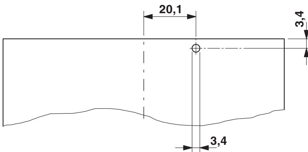
Bohrplan/Lötpadgeometrie
