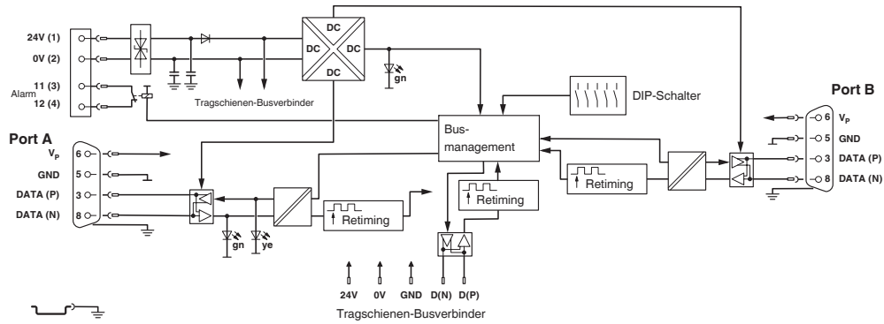
Blockschaltbild
