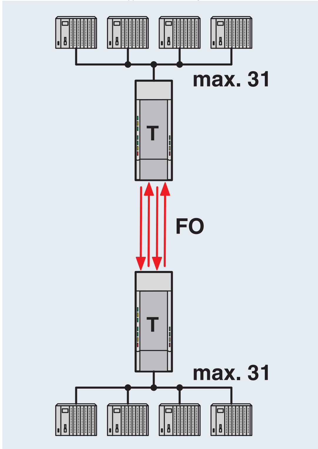
Redundante Punkt-zu-Punkt-Verbindung
