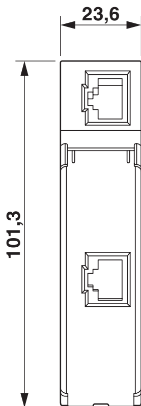
Gehäuseabmessungen
