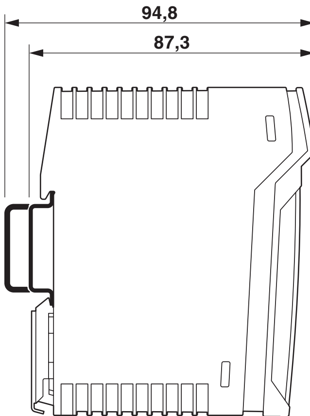
Maßzeichnung
