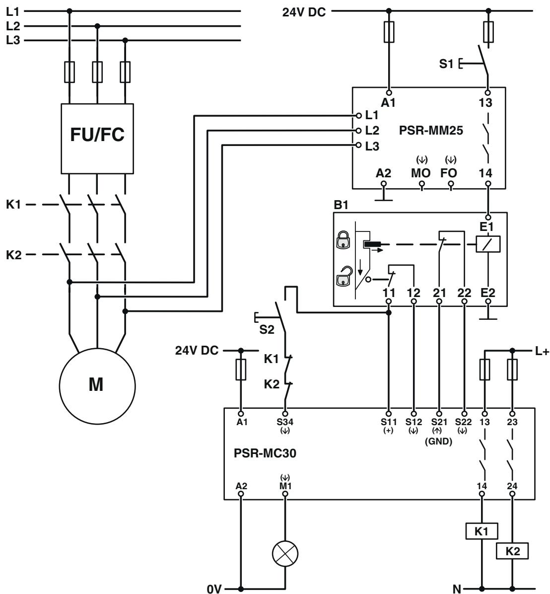
Schaltplan
