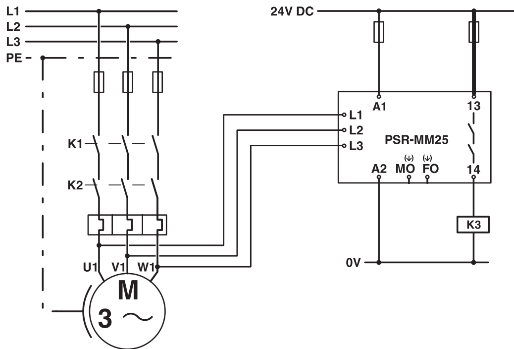
Schaltplan
